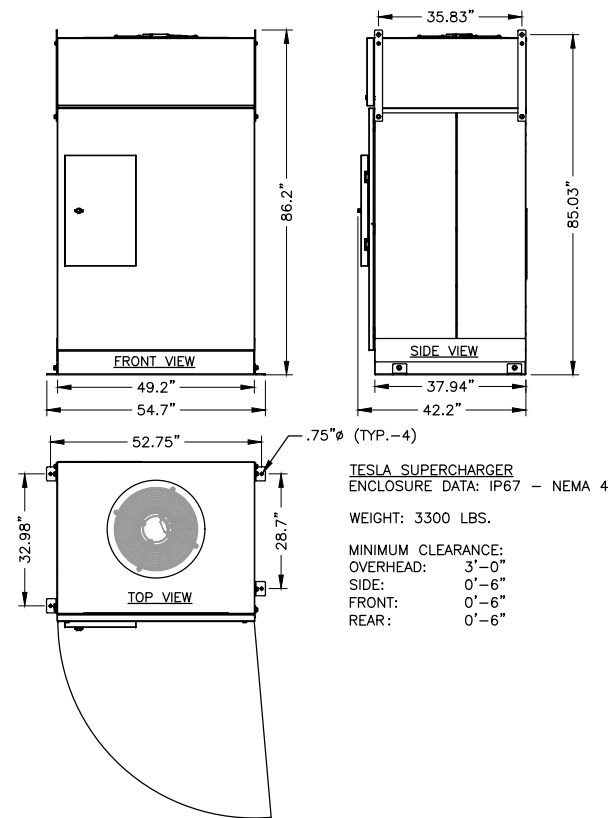
TESLA SUPERCHARGER CABINET DETAIL SCALE: N.T.S.
