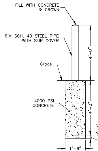
CONCRETE BOLLARD DETAIL SCALE: N.T.S.
